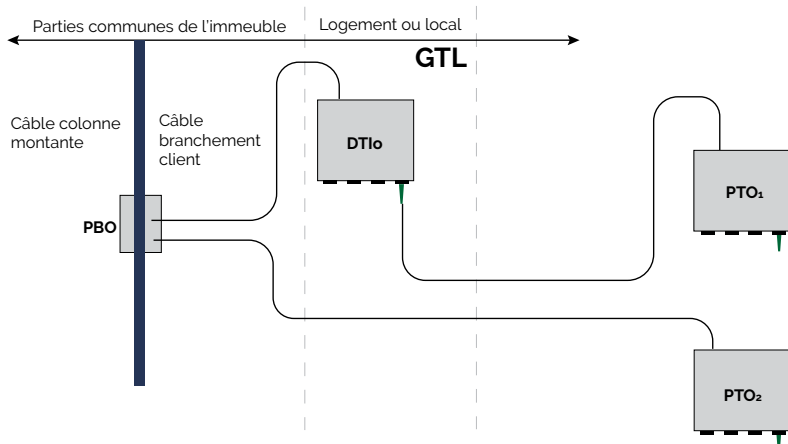
Fig. 05 | Emplacement du DTIo et de la PTO dans le logement
