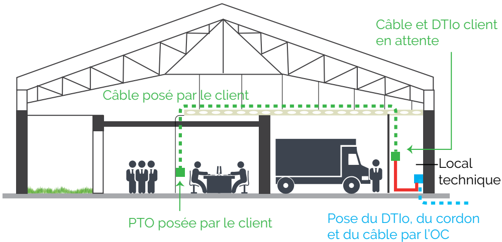
Fig. 48 | Reprise du câble client par jarretière : cas N°3
