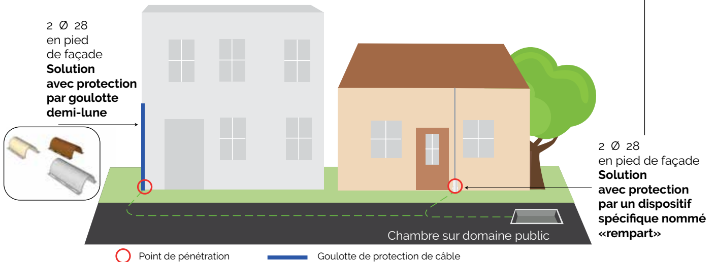
Fig. 40 | Protections aéro-souterraines
