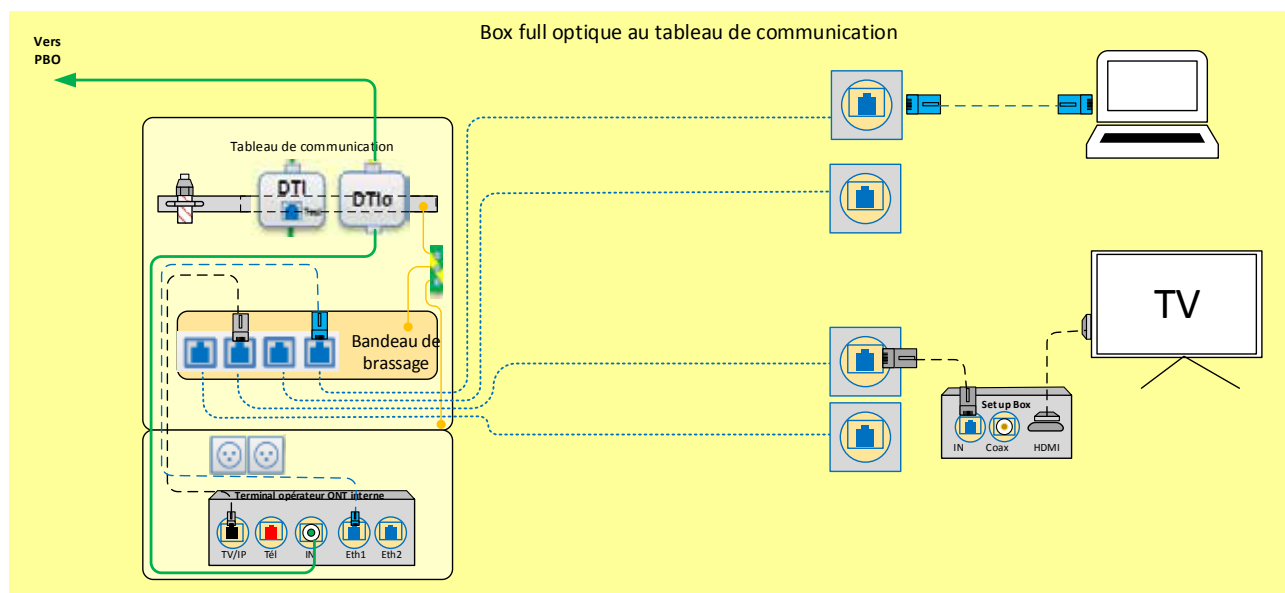
Fig. 65 | Installation avec Box (ONT intégré) dans le tableau de communication
