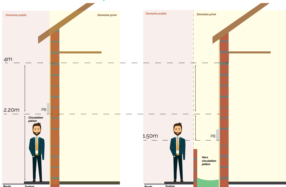
Fig. 86 | Hauteur minimale du PBO sur façade
