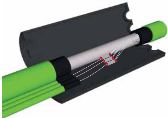
Fig. 97 | Boitier de jonction pour solution micro-conduits
