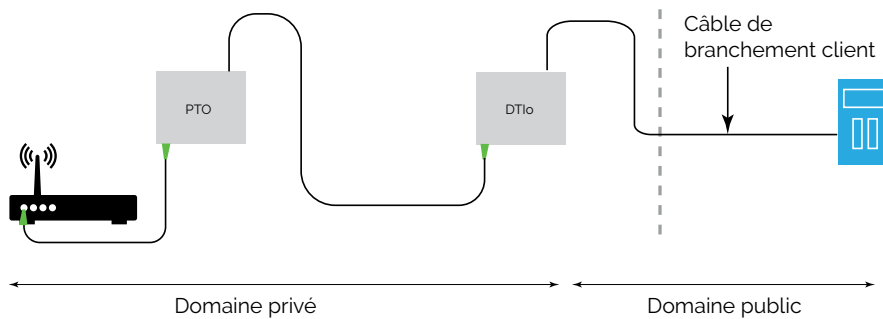
Fig. 48 | Reprise du câble client par jarretière : cas N°3
