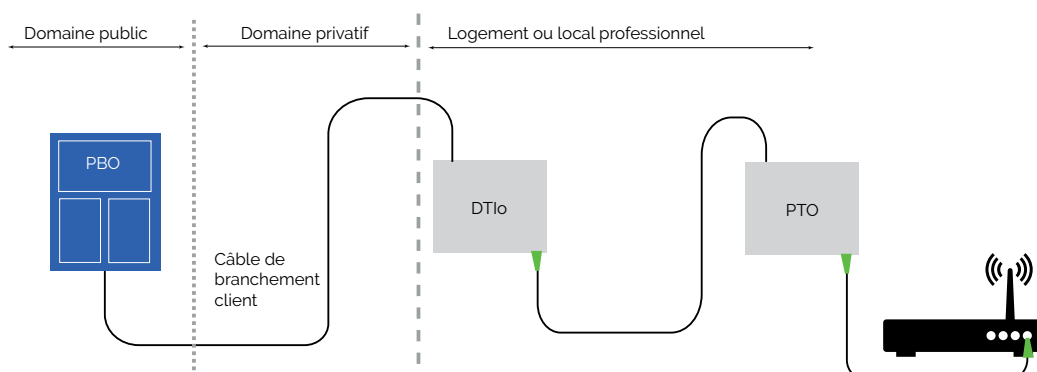
Fig. 63 | installation avec déport à partir d'un DTIo (à privilégier)
