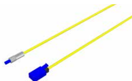
Fig. 96 | unité mono-fibre « pré-ferrulée » pour soufflage
