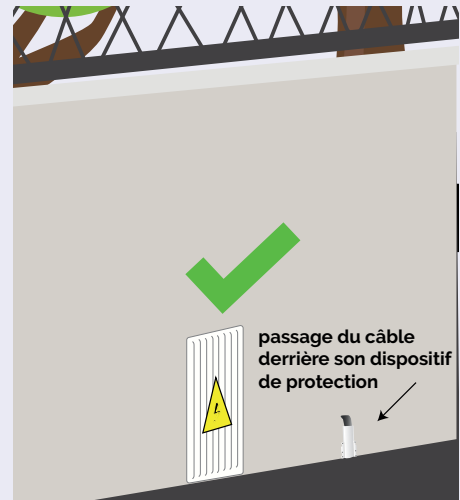
Fig. 21 | Cas d'une colonne rampante extérieure conforme
