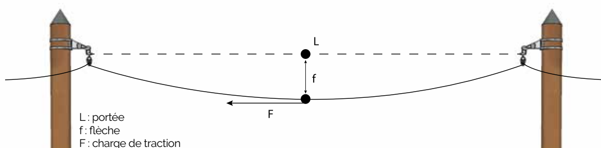
Fig. 29 | Calcul théorique d'une flèche
